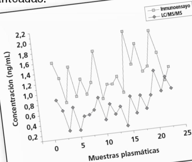
Figura 1. Concentración plasmática de la digoxina (ng/mL) analizada por inmunoensayo y por LC-MS/MS de 15 pacientes del Ambulatorio de Insuficiencia Cardíaca del HC-UFG (n = 23).
